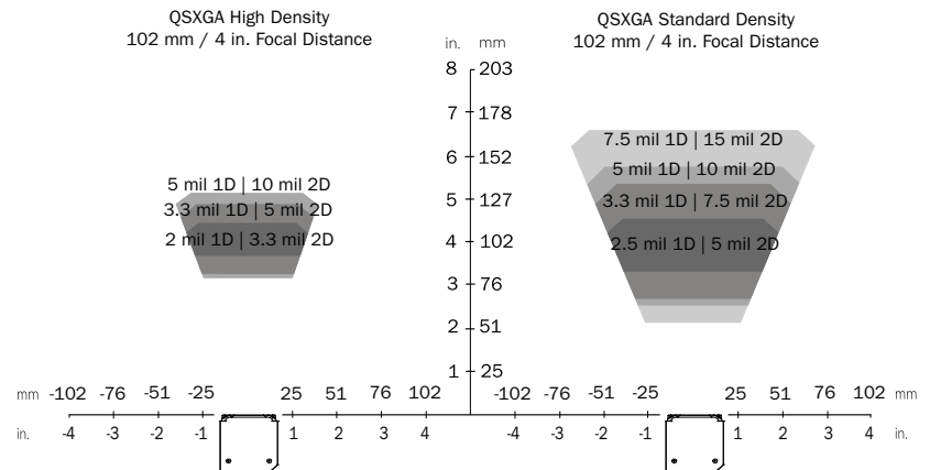
QXSGA 传感器：读取范围样例
